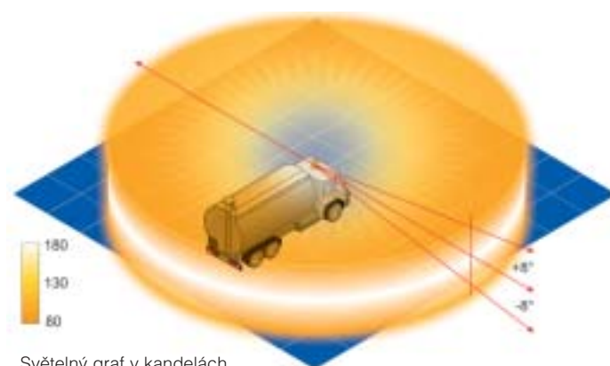
Světelný graf v kandelách
